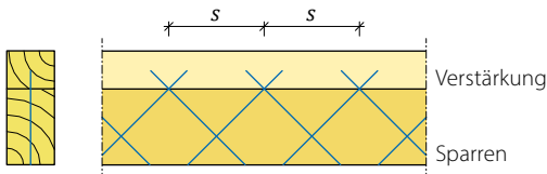
Bild 6. Mögliche Schraubenlagen bei gekreuzten Schraubenpaaren
