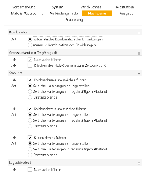
Bild 9. Eingabe „Nachweise“ – Grenzzustand der Tragfähigkeit
