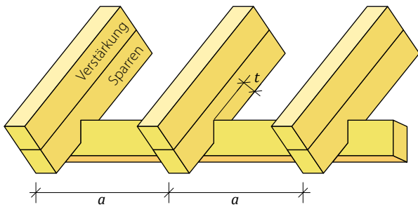
Bild 8. Querschnittschwächung an den Auflagern
