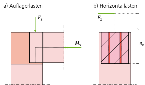
Bild 9. Belastung (Prinzipiskizze)
