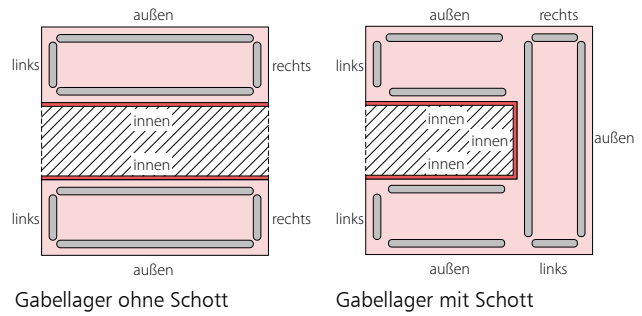
Bild 12. Manuelle Bewehrungsanordnung, Auswahl Lagen (Prinzipische Skizzen)
