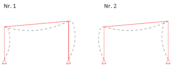
Bild 7. Pultdachrahmen mit Schiefstellung und Vorkrümmung
