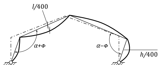
Bild 8. Imperfektionen im Holzbau nach EC 5
