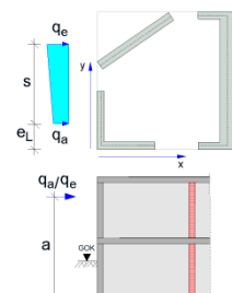
horizontale Trapezlast
