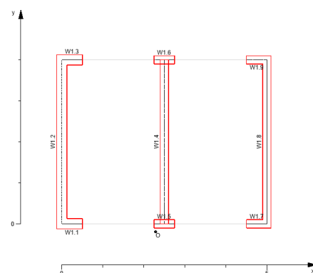
Bild 4. System „Beispiel: Aussteifungskern-Aufzugsschacht“
