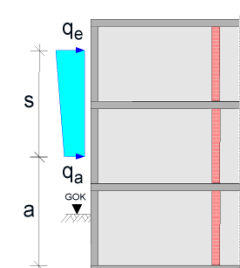
vertikale Trapezlast
