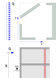
horizontale Gleichlast
