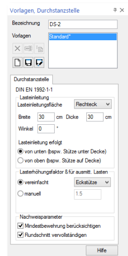
Bild 7. Eigenschaften der Durchstanzstelle
