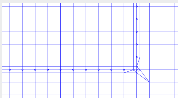
Bild 5. FE-Netz mit „Netzanpassung am Anschnitt“
