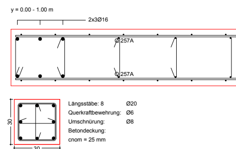
Bild 11. Beispielausgabe umschnürte Wand- und Stützenenden
