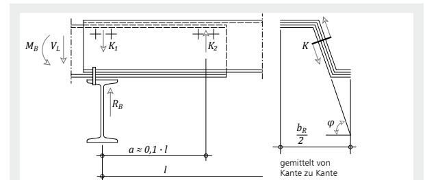
Bild 7. a) Überkragendes Ende der Profiltafeln liegt unten
