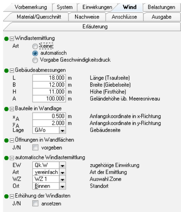
Bild 2. Definitionen zu Windlasten
