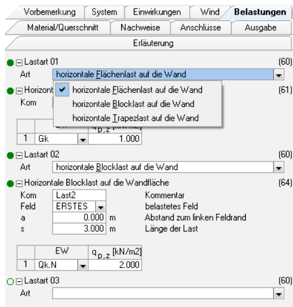
Bild 3. Definitionen im Kapitel „Belastung“
