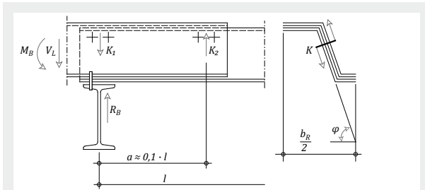
Bild 7. b) Überkragendes Ende der Profiltafeln liegt oben
