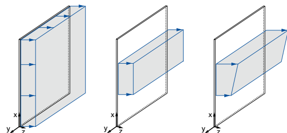
Bild 4. Mögliche Lastdefinitionen: Gleich-, Block- und Trapezlast
