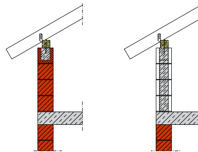
Bild 2. Drempel – Schnitte durch Mauerwerk und Kragstütze
