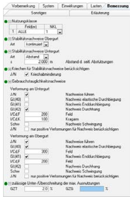
Bild 3. Eingaberegister „Bemessung“
