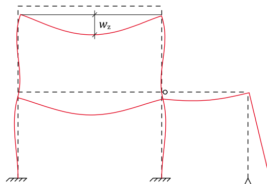
Nachweis Durchbiegung Einzelstäbe
