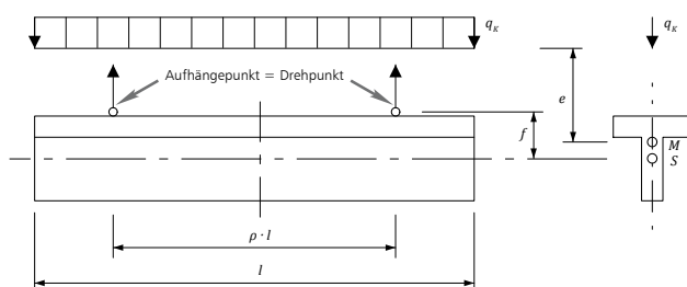
Berechnungsmodell für den kippgefährdeten, aufgehängten Träger nach Lebel
