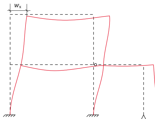
Nachweis Kopfverschiebungen
